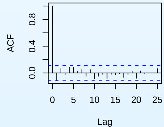
AR-HMM
