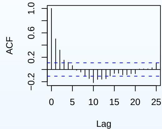
Serfling
