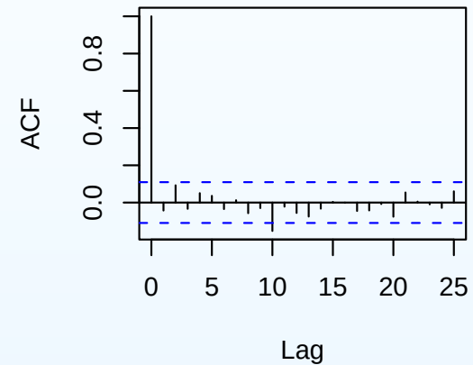
AR-HMM
